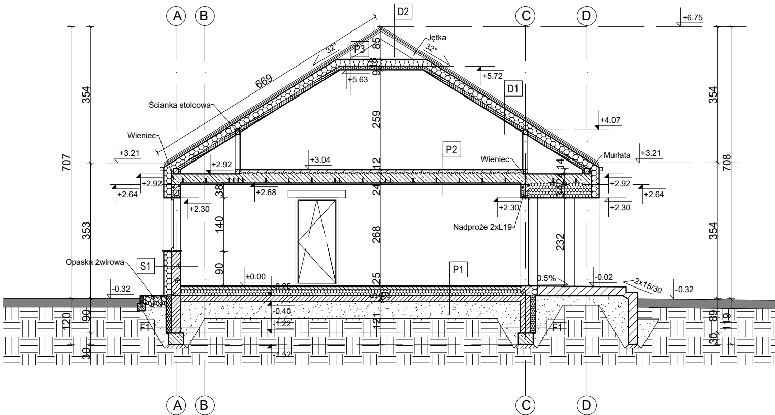
Przekrój A3-A3
